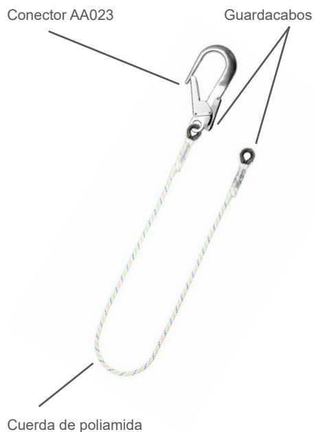
Eslinga simple fija 610104-015
