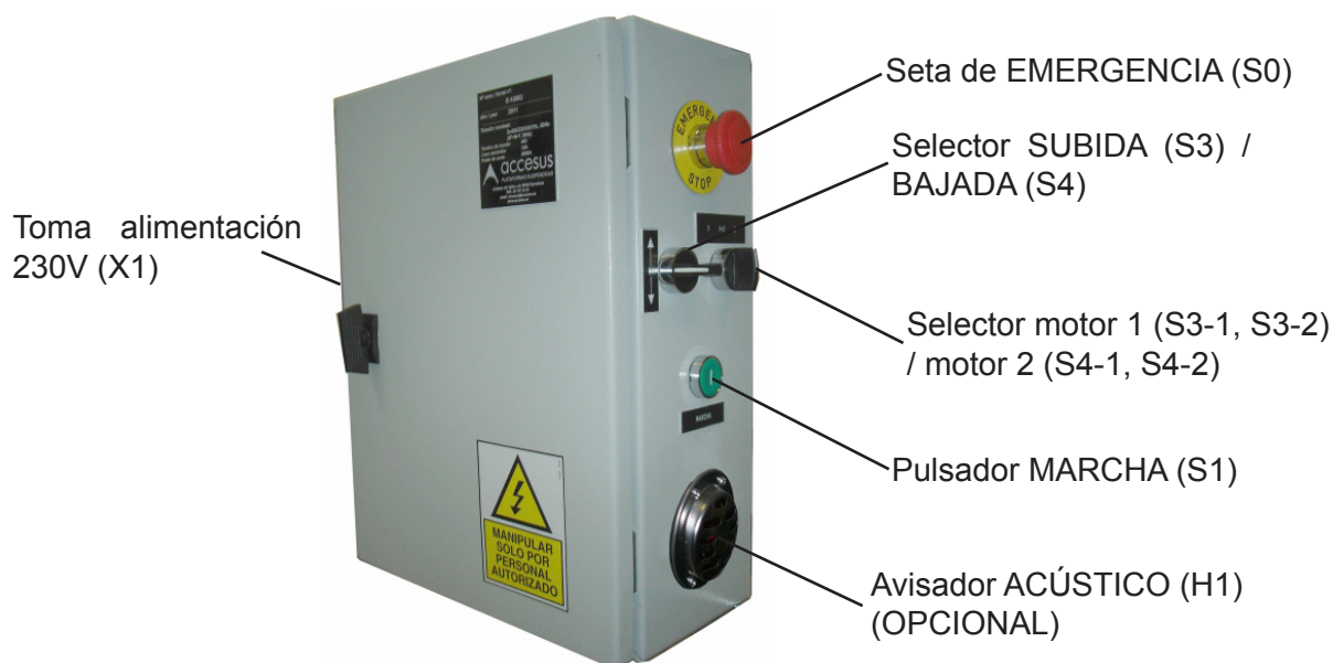
Armario eléctrico
