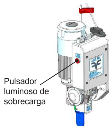
Elevador e.lift501
