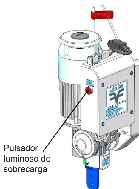
Elevador e.lift501
