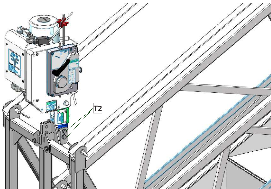
Posición interna
