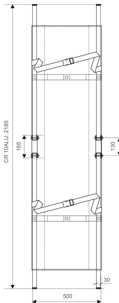
Camilla CR 10ALU cotas
