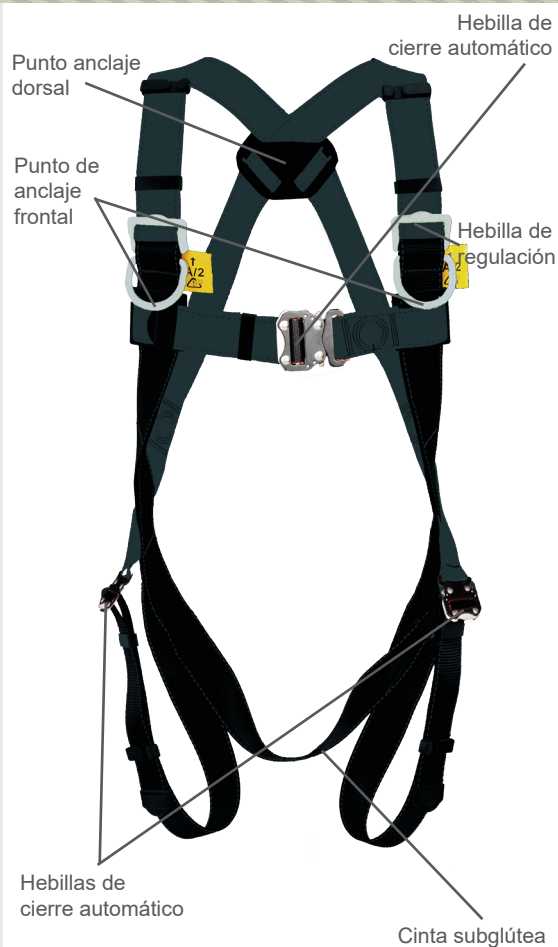
Arnés anticaídas de seguridad A40BC BLACK
