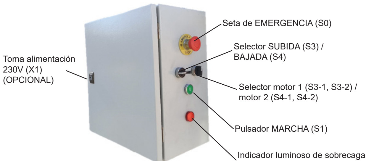
Armario eléctrico
